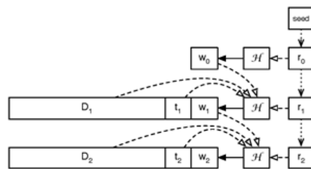
Abbildung 2020 – Chained Transaction Log
